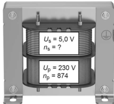
schematische weergave van de transformator
