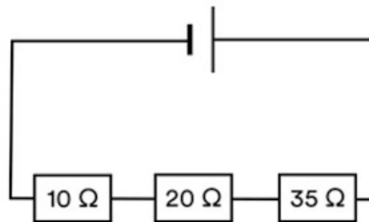
Serie schakeling
